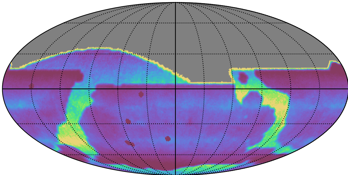
ddf_acor_sf25_lsf30_lsr10_v3.4_10yrs : DCRprecision
