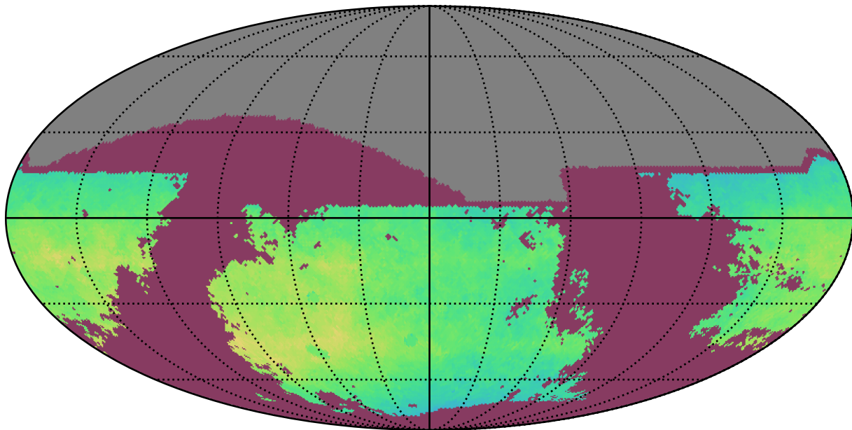
ddf_acor_sf20_lsf40_lsr50_v3.4_10yrs i: NgalScale
