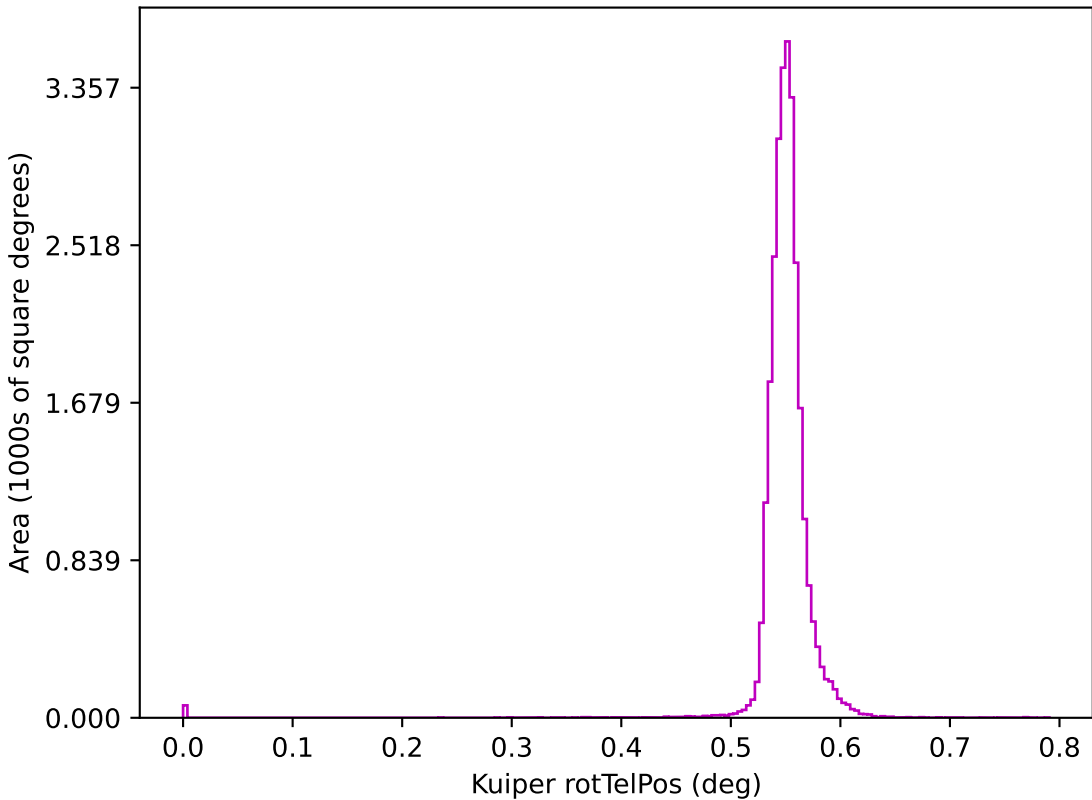
ddf_acor_sf20_lsf40_lsr50_v3.4_10yrs z: Kuiper rotTelPos
