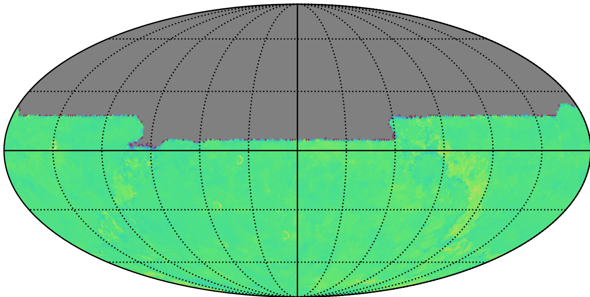
ddf_acor_sf20_lsf40_lsr50_v3.4_10yrs u: Kuiper rotTelPos
