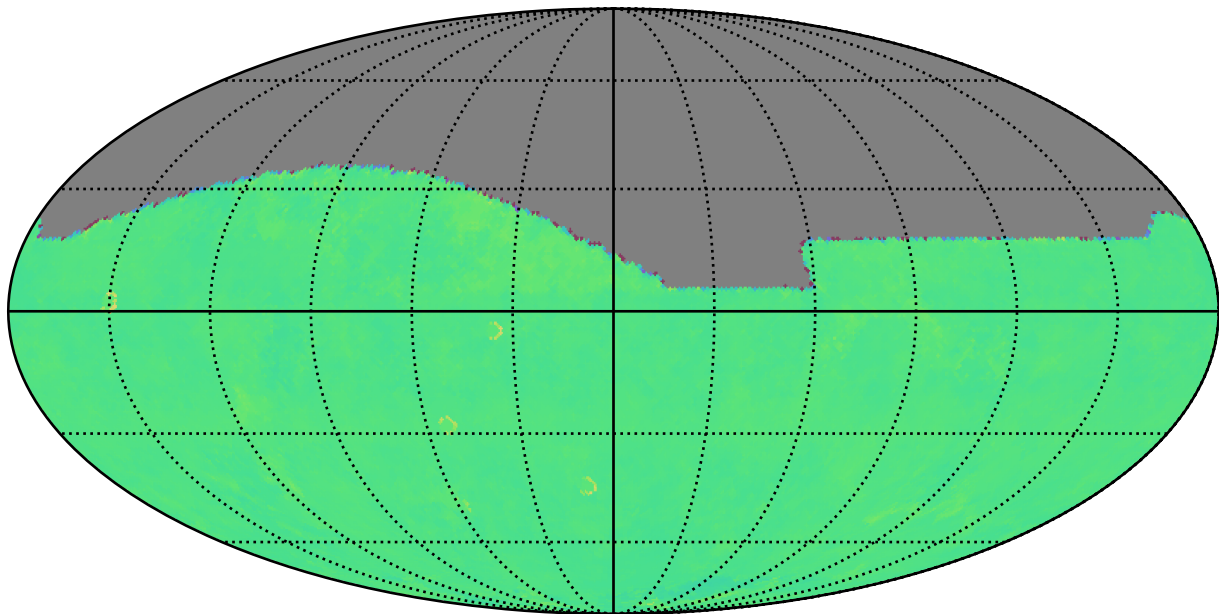
ddf_acor_sf20_lsf40_lsr50_v3.4_10yrs i: Kuiper rotTelPos
