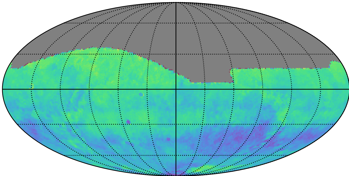
ddf_acor_sf20_lsf40_lsr50_v3.4_10yrs i: Kuiper rotSkyPos
