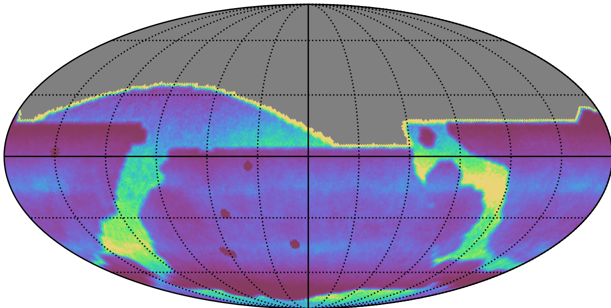
ddf_acor_sf20_lsf40_lsr50_v3.4_10yrs : DCRprecision
