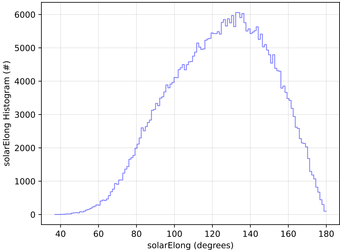
ddf_acor_sf20_lsf40_lsr50_v3.4_10yrs All sky y band: solarElong Histogram
