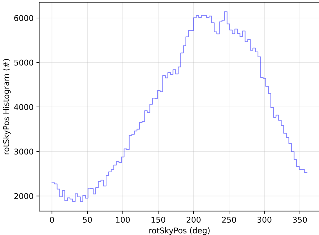
ddf_acor_sf20_lsf40_lsr50_v3.4_10yrs All sky y band: rotSkyPos Histogram
