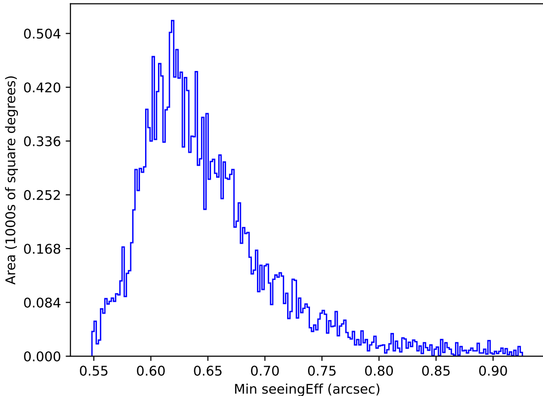
ddf_acor_sf20_lsf40_lsr50_v3.4_10yrs All sky y band: Min seeingEff
