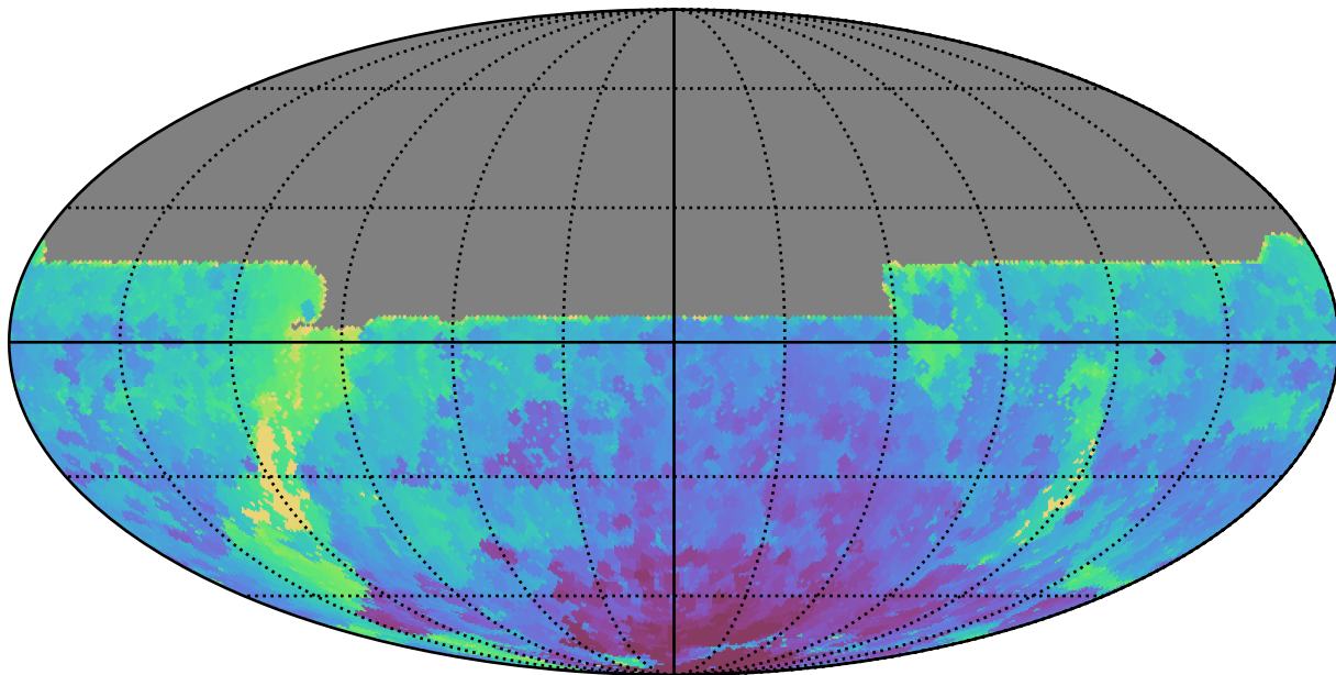
ddf_acor_sf20_lsf40_lsr50_v3.4_10yrs All sky y band: Min HA
