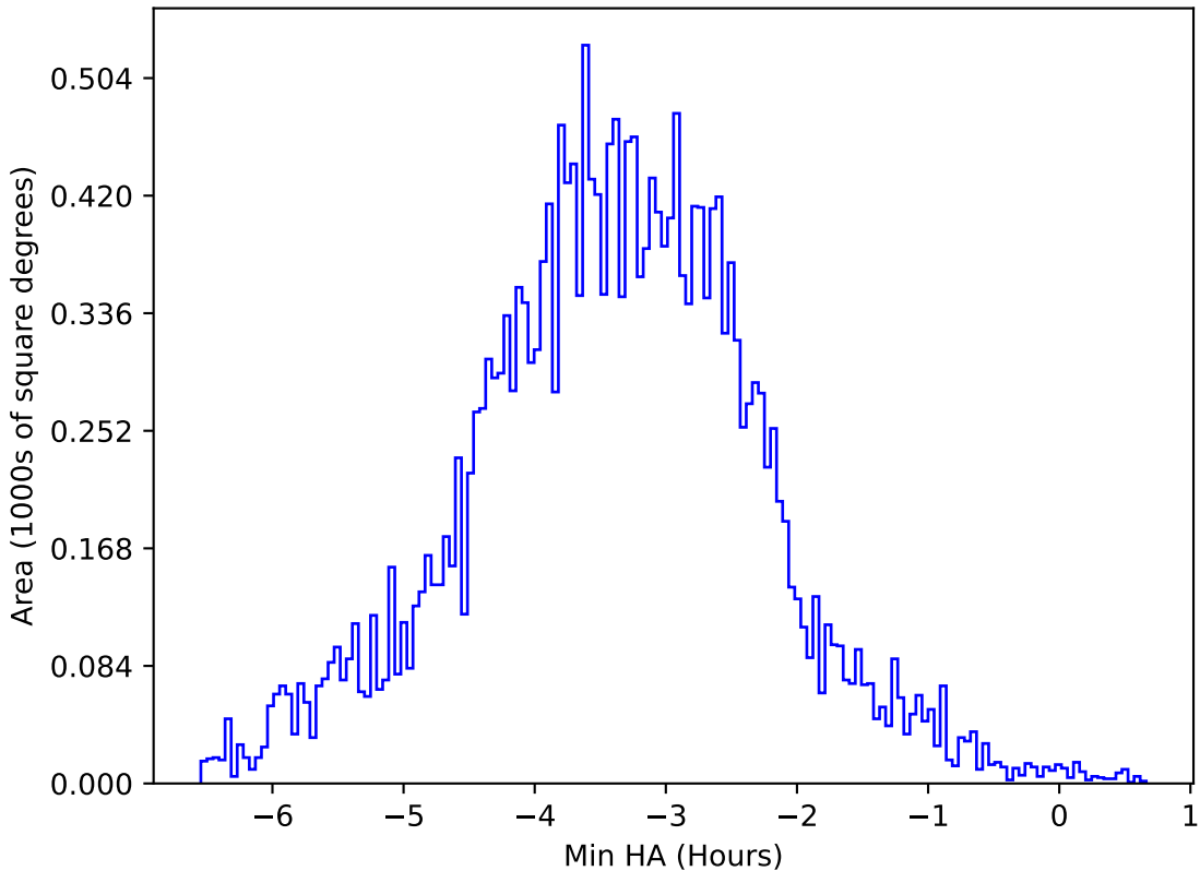
ddf_acor_sf20_ls40_lsr50_v3.4_10yrs All sky y band: Min HA
