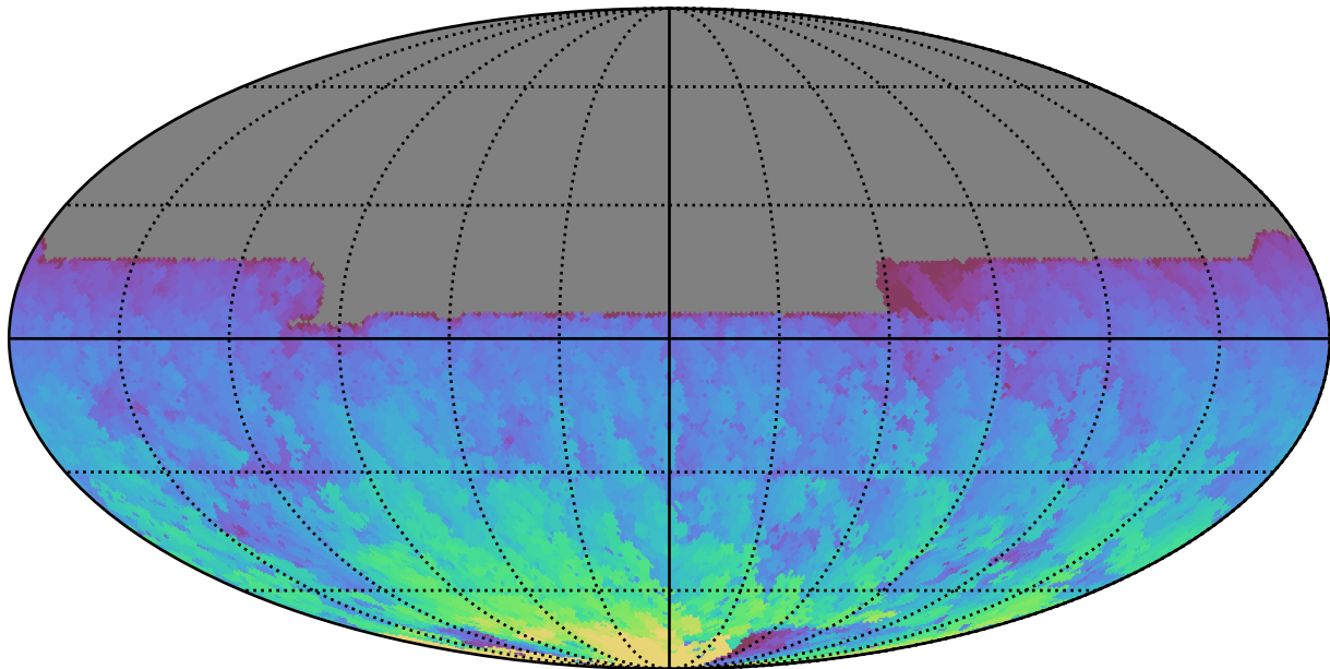
ddf_acor_sf20_lsf40_lsr50_v3.4_10yrs All sky y band: Max HA
