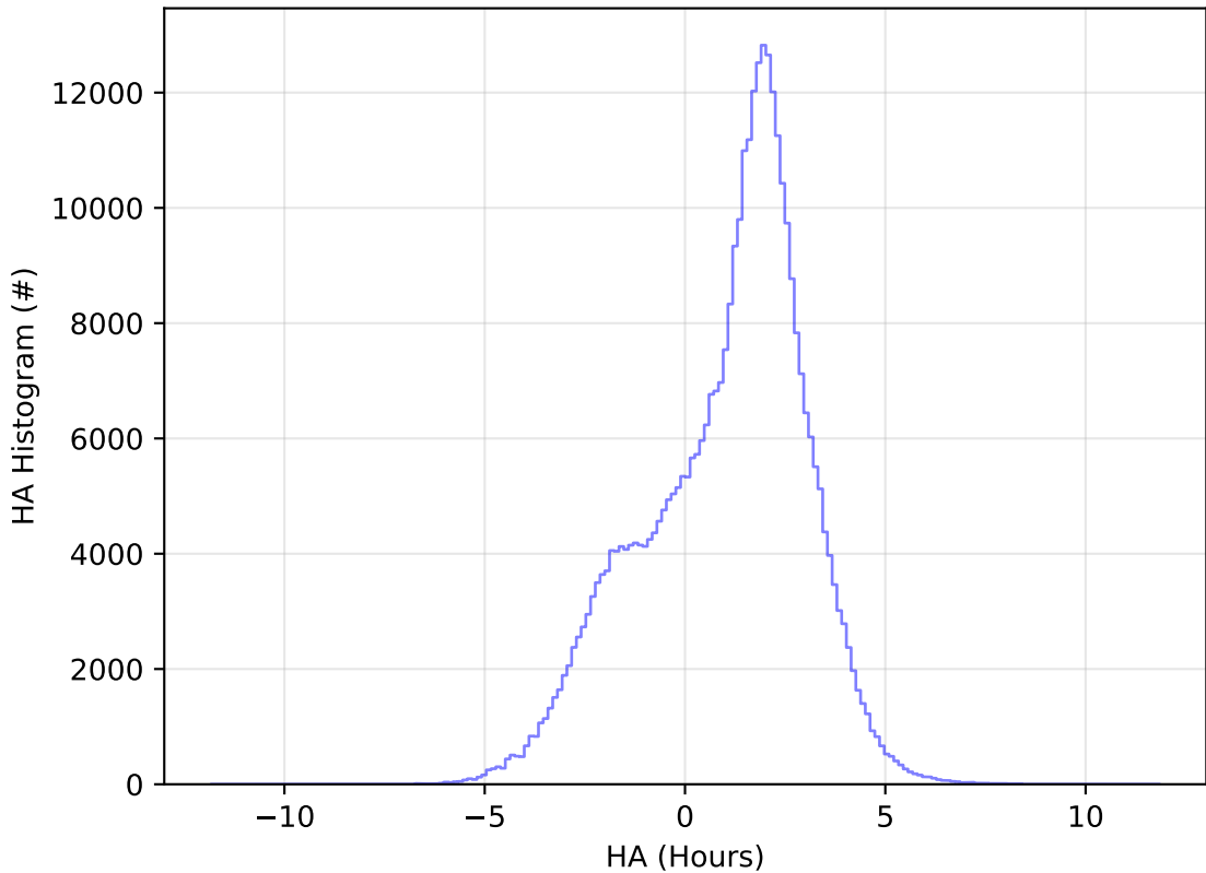
ddf_acor_sf20_lsf40_lsr50_v3.4_10yrs All sky y band: HA Histogram
