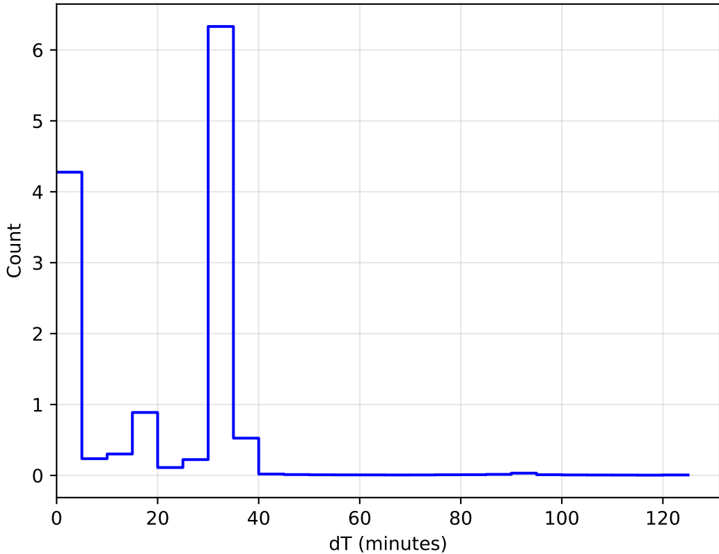
ddf_acor_sf20_lsf40_lsr50_v3.4_10yrs All sky: DeltaT Histogram
