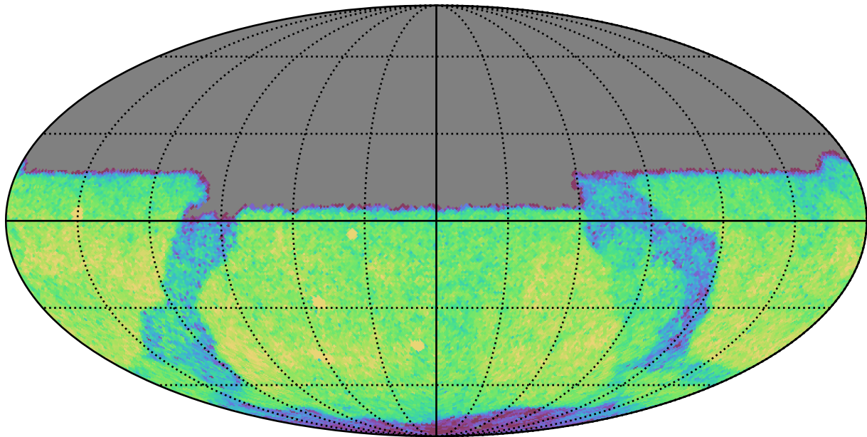
ddf_acor_sf20_lsf40_lsr50_v3.4_10yrs Yr 1 y band: CoaddM5
