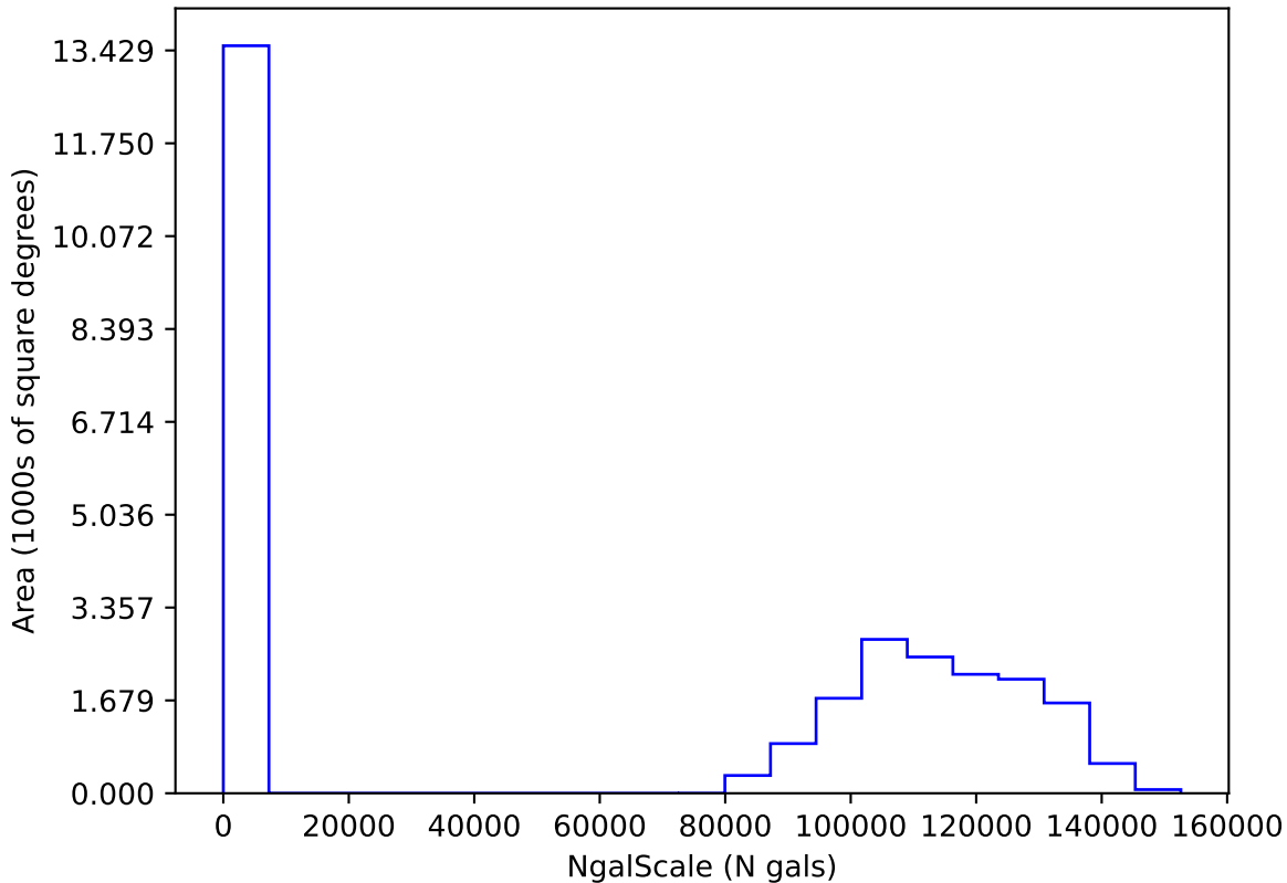
ddf_acor_sf20_lsf40_lsr20_v3.4_10yrs i: NgalScale
