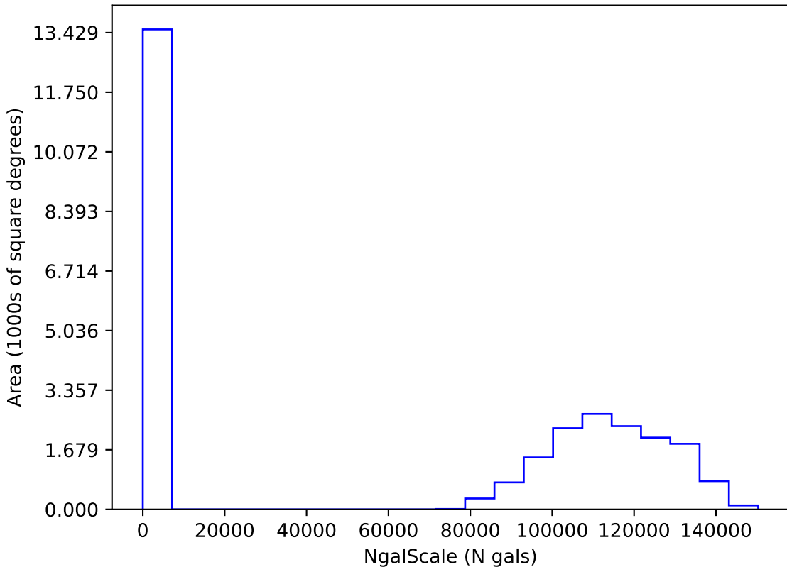
ddf_acor_sf20_lsf40_lsr10_v3.4_10yrs i: NgalScale
