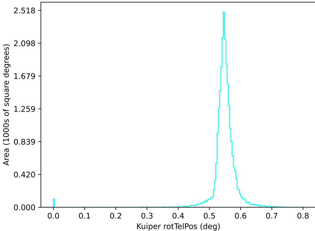
ddf_acor_sf20_ls40_lsr10_v3.4_10yrs u: Kuiper rotTelPos
