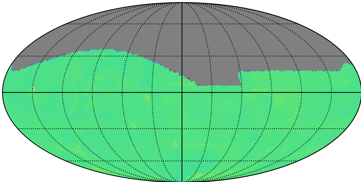
ddf_acor_sf20_lsf40_lsr10_v3.4_10yrs r: Kuiper rotTelPos
