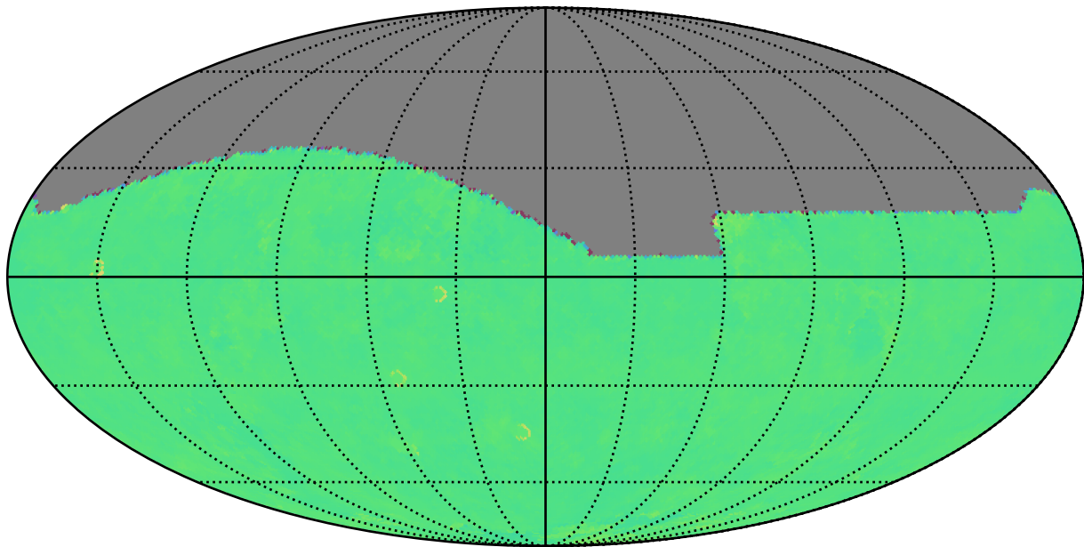
ddf_acor_sf20_lsf40_lsr10_v3.4_10yrs i: Kuiper rotTelPos
