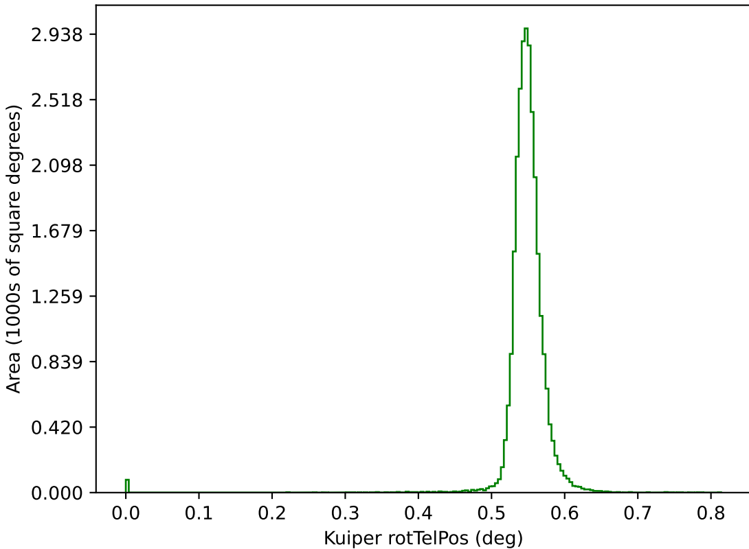
ddf_acor_sf20_lsf40_lsr10_v3.4_10yrs g: Kuiper rotTelPos
