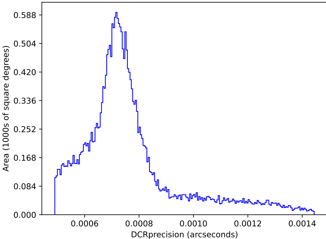
ddf_acor_sf20_ls40_lsr10_v3.4_10yrs : DCRprecision
