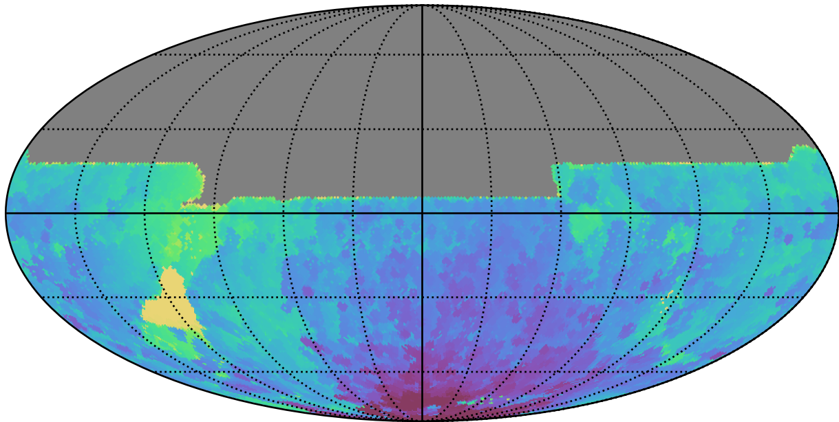
ddf_acor_sf20_lsf40_lsr10_v3.4_10yrs All sky y band: Min HA
