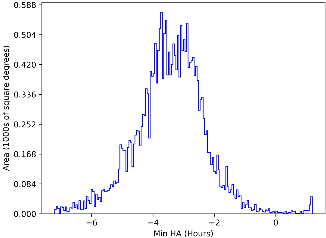
ddf_acor_sf20_lsf40_lsr10_v3.4_10yrs All sky y band: Min HA
