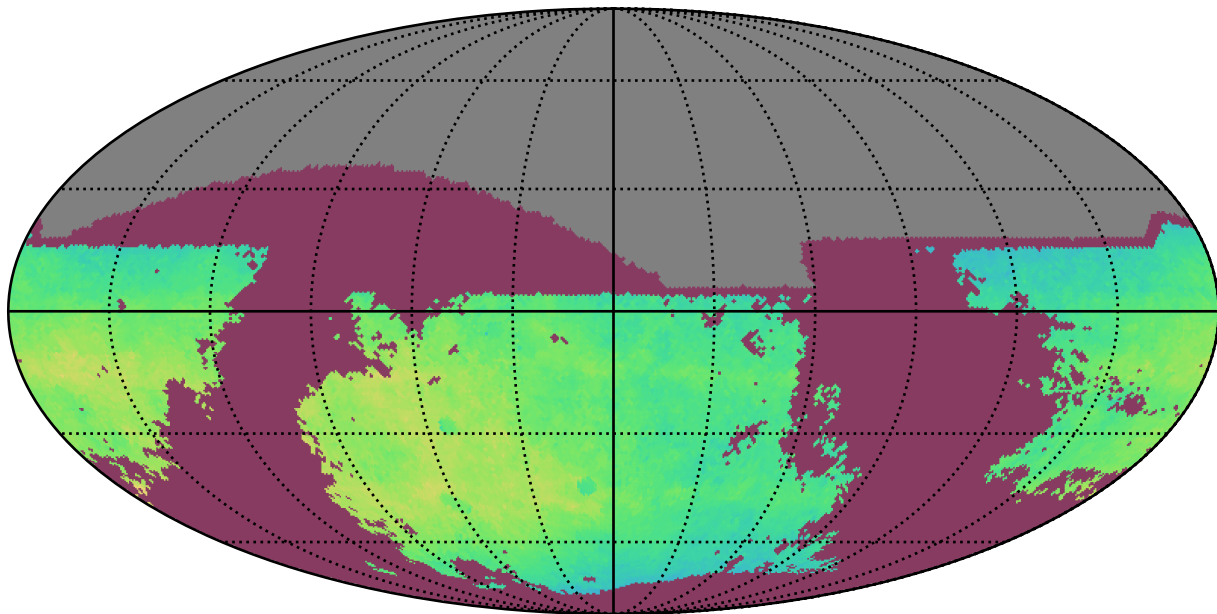
ddf_acor_sf20_lsf30_lsr50_v3.4_10yrs i: NgalScale
