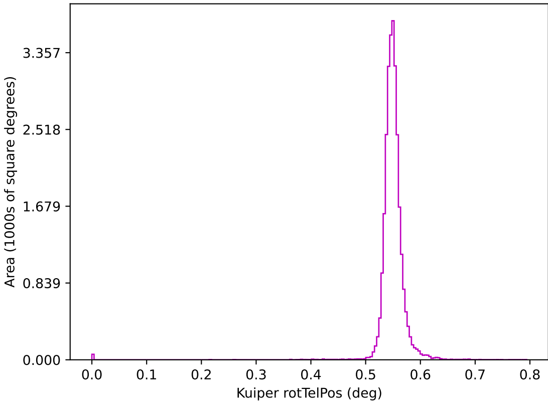
ddf_acor_sf20_lsf30_lsr50_v3.4_10yrs z: Kuiper rotTelPos
