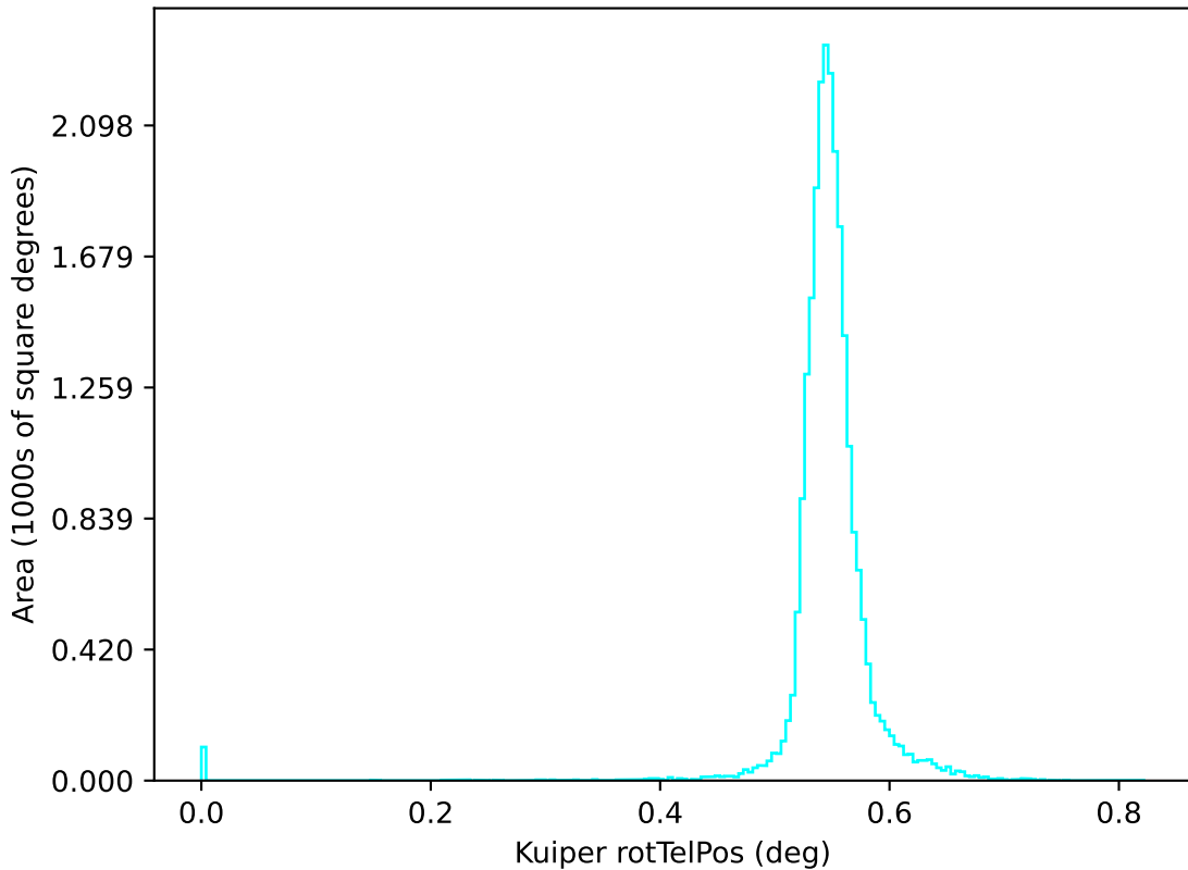
ddf_acor_sf20_ls30_lsr50_v3.4_10yrs u: Kuiper rotTelPos
