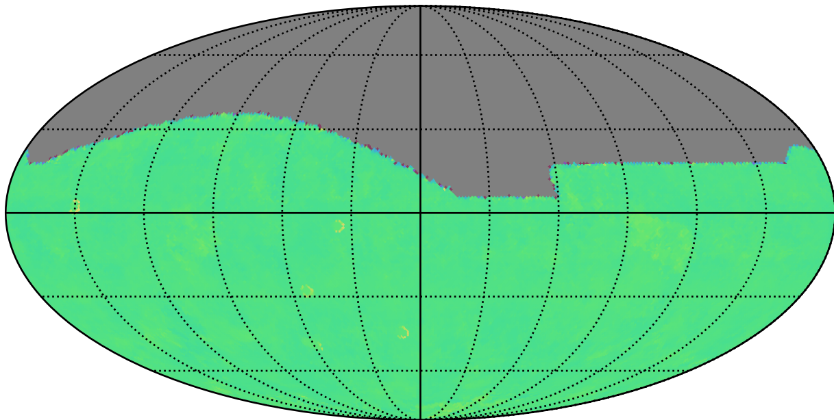
ddf_acor_sf20_lsf30_lsr50_v3.4_10yrs i: Kuiper rotTelPos
