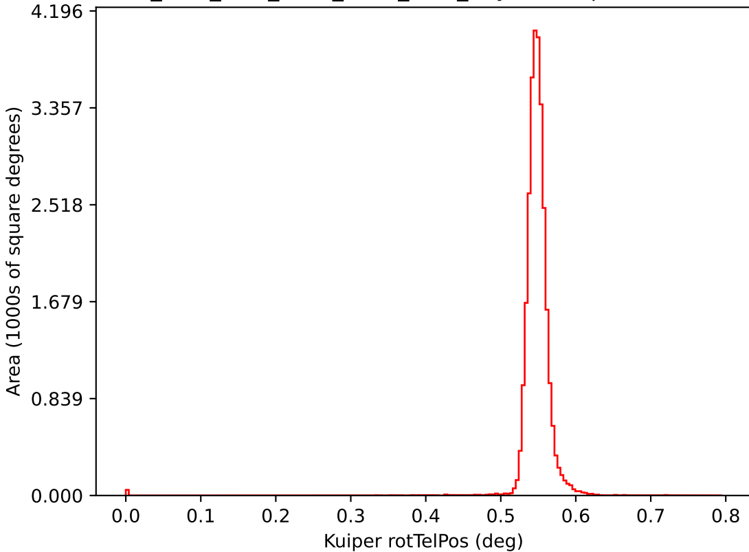
ddf_acor_sf20_lsf30_lsr50_v3.4_10yrs i: Kuiper rotTelPos
