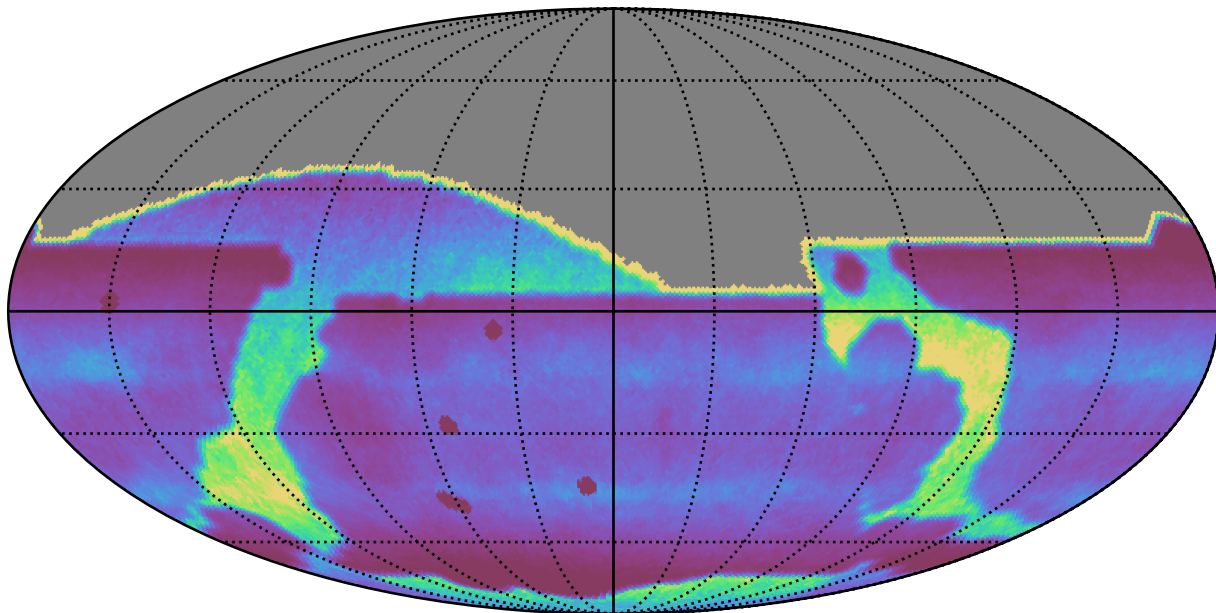
ddf_acor_sf20_lsf30_lsr50_v3.4_10yrs : DCRprecision
