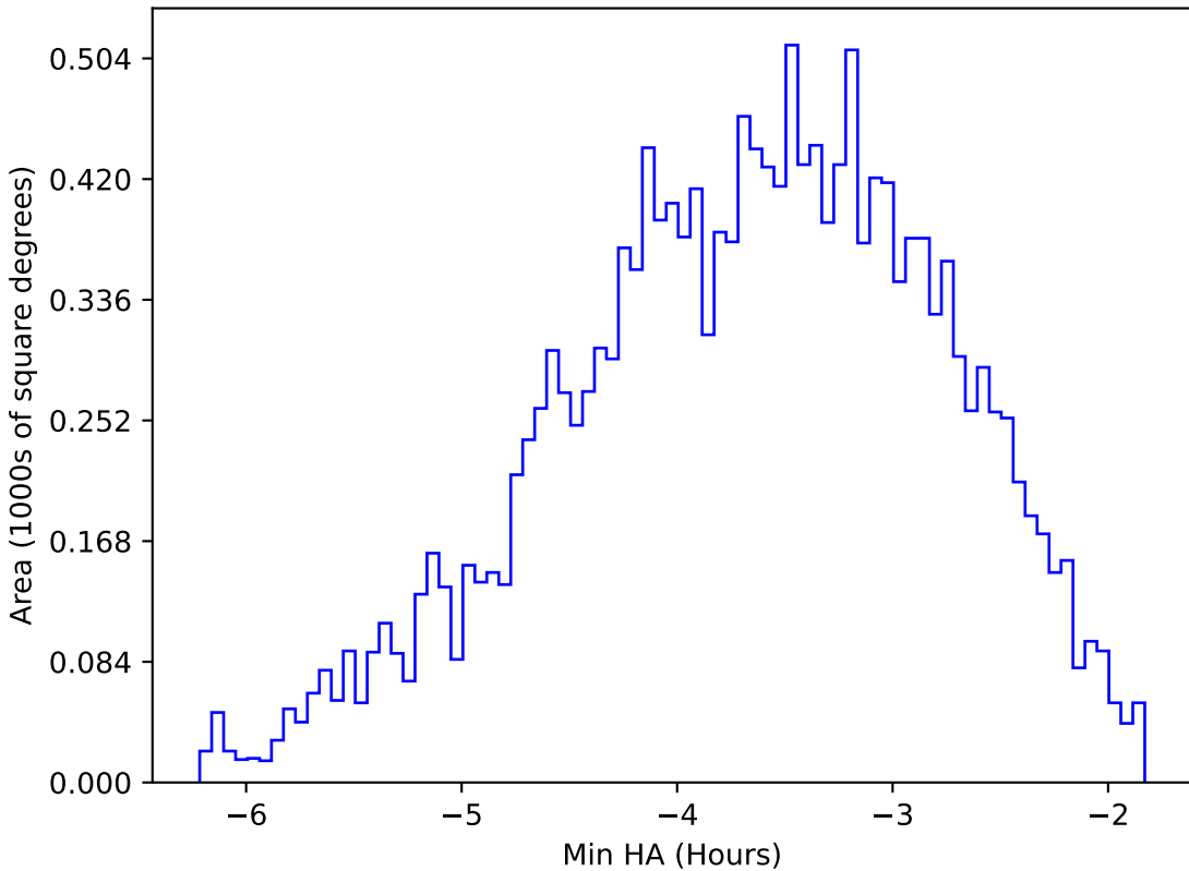
ddf_acor_sf20_lsf30_lsr50_v3.4_10yrs WFD y band: Min HA
