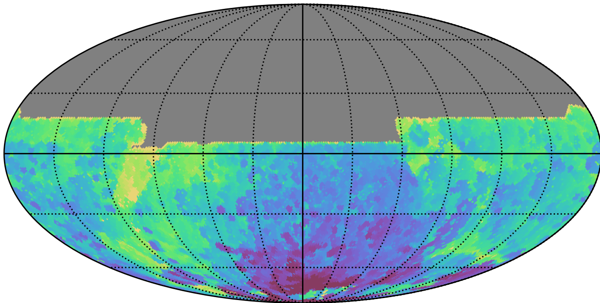
ddf_acor_sf20_lsf30_lsr50_v3.4_10yrs All sky y band: Min HA
