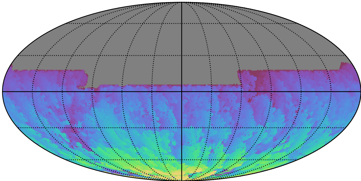
ddf_acor_sf20_lsf30_lsr50_v3.4_10yrs All sky y band: Max HA
