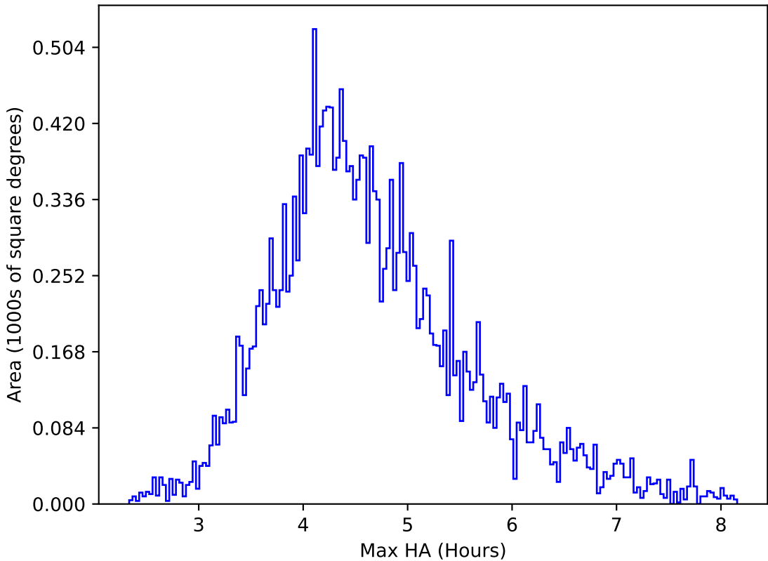
ddf_acor_sf20_lsf30_lsr50_v3.4_10yrs All sky y band: Max HA
