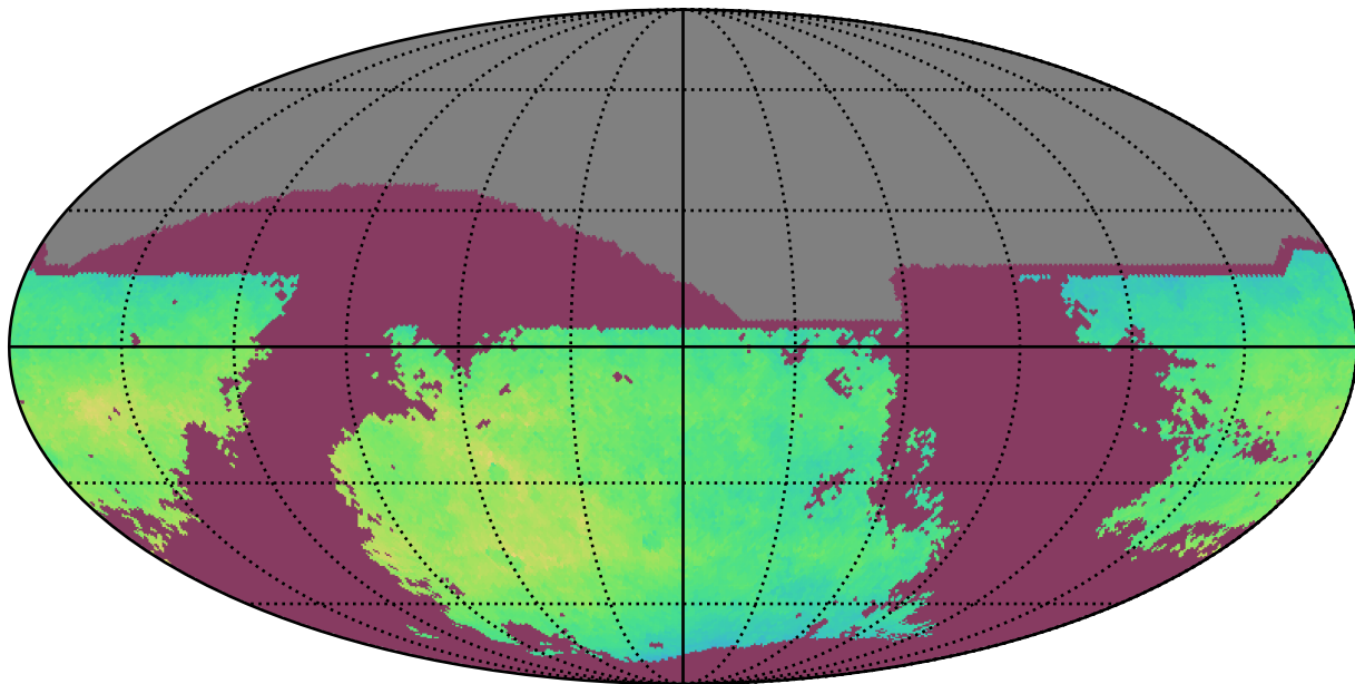
ddf_acor_sf20_lsf30_lsr20_v3.4_10yrs i: NgalScale
