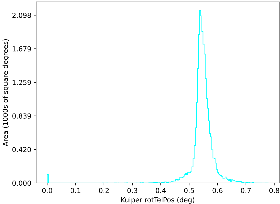
ddf_acor_sf20_lsf30_lsr20_v3.4_10yrs u: Kuiper rotTelPos
