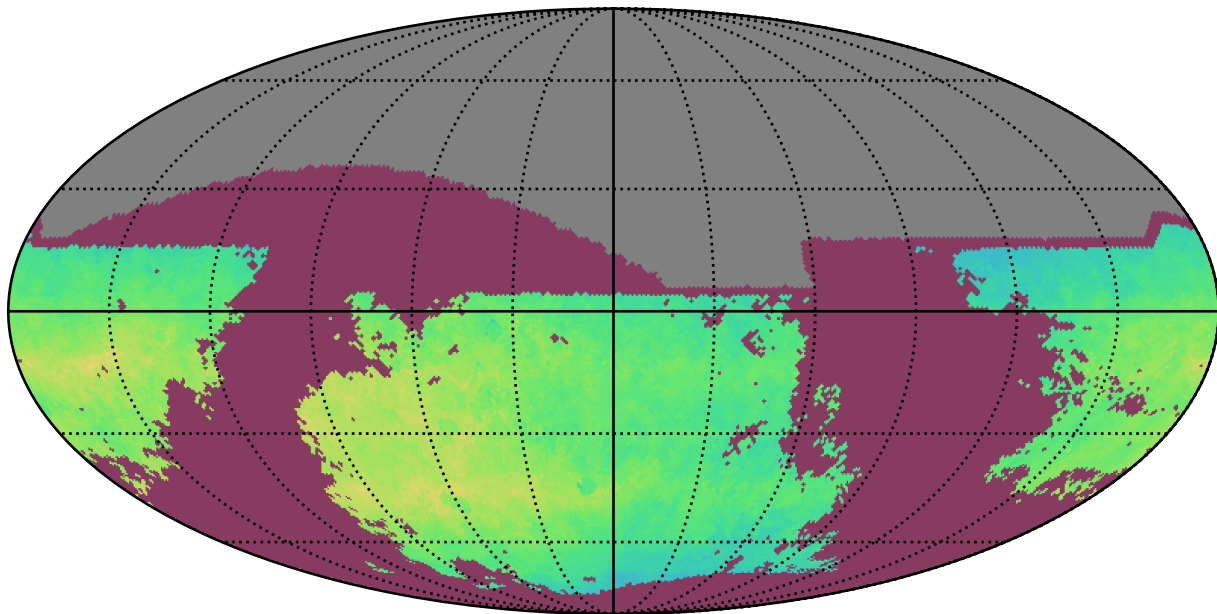
ddf_acor_sf20_lsf30_lsr10_v3.4_10yrs i: NgalScale
