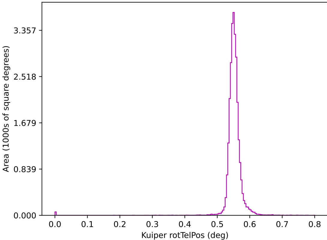
ddf_acor_sf20_lsf30_lsr10_v3.4_10yrs z: Kuiper rotTelPos
