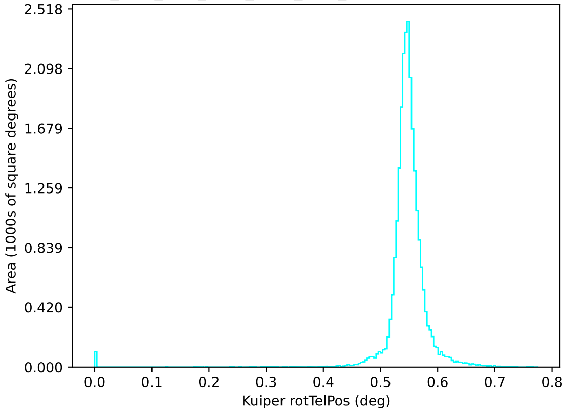
ddf_acor_sf20_ls30_lsr10_v3.4_10yrs u: Kuiper rotTelPos
