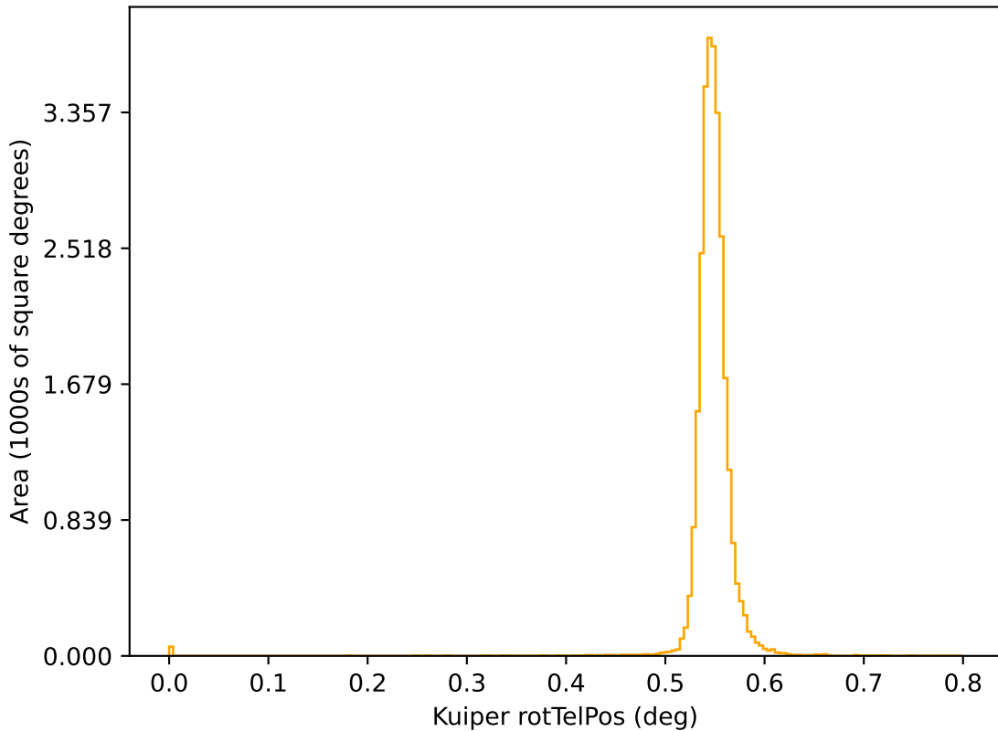
ddf_acor_sf20_lsf30_lsr10_v3.4_10yrs r: Kuiper rotTelPos
