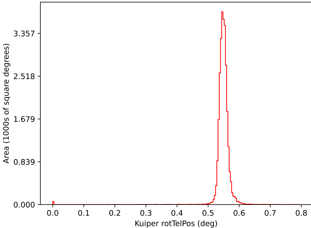
ddf_acor_sf20_lsf30_lsr10_v3.4_10yrs i: Kuiper rotTelPos
