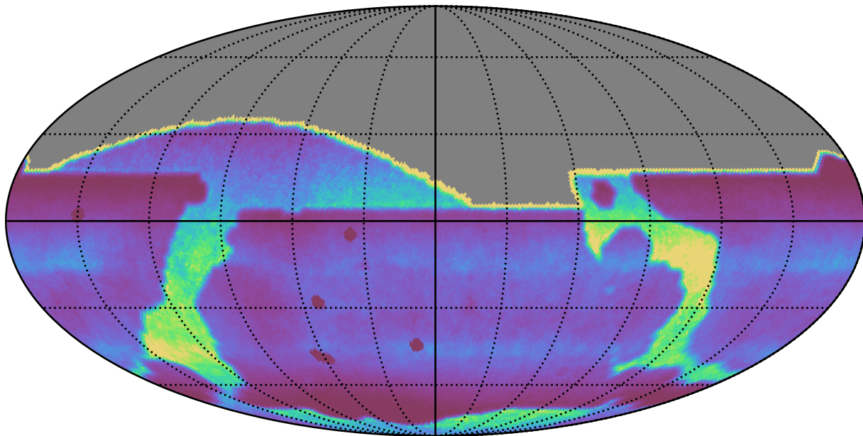
ddf_acor_sf20_lsf30_lsr10_v3.4_10yrs : DCRprecision
