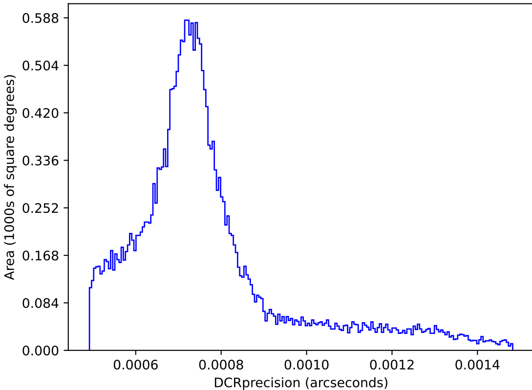
ddf_acor_sf20_ls30_lsr10_v3.4_10yrs : DCRprecision
