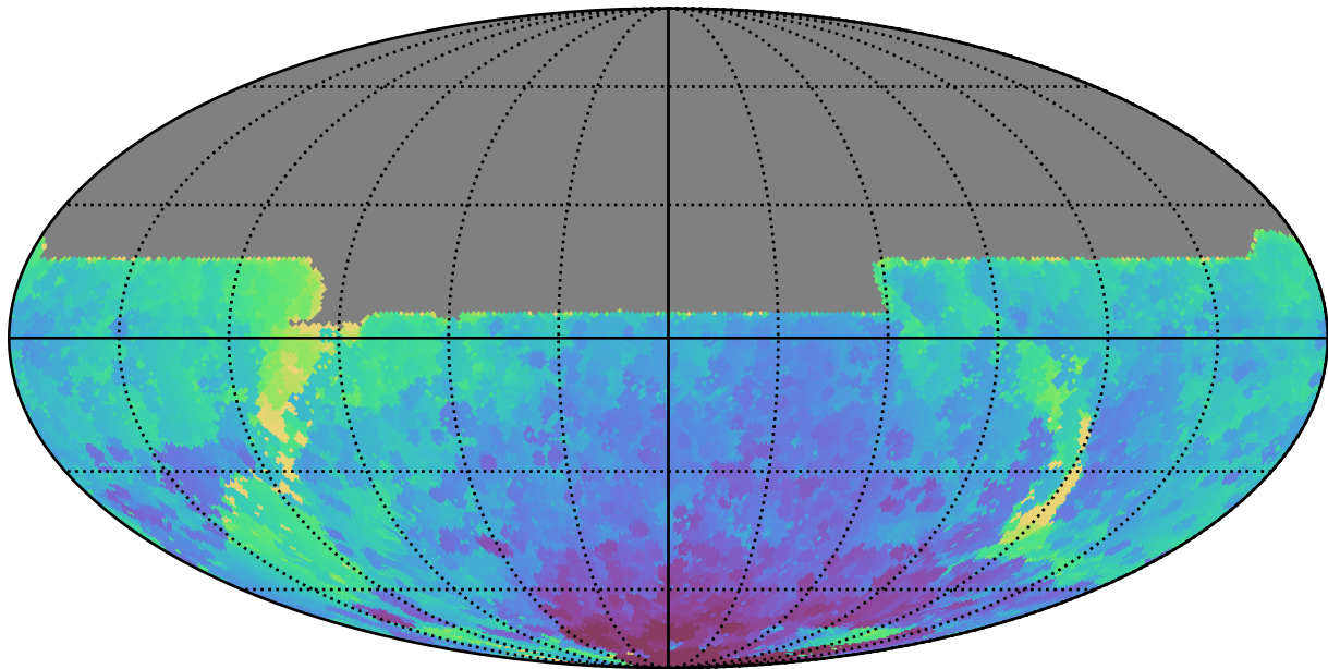
ddf_acor_sf20_lsf30_lsr10_v3.4_10yrs All sky y band: Min HA
