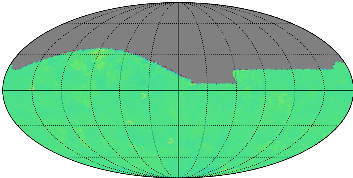
ddf_acor_sf20_lsf0_lsr0_v3.4_10yrs z: Kuiper rotTelPos
