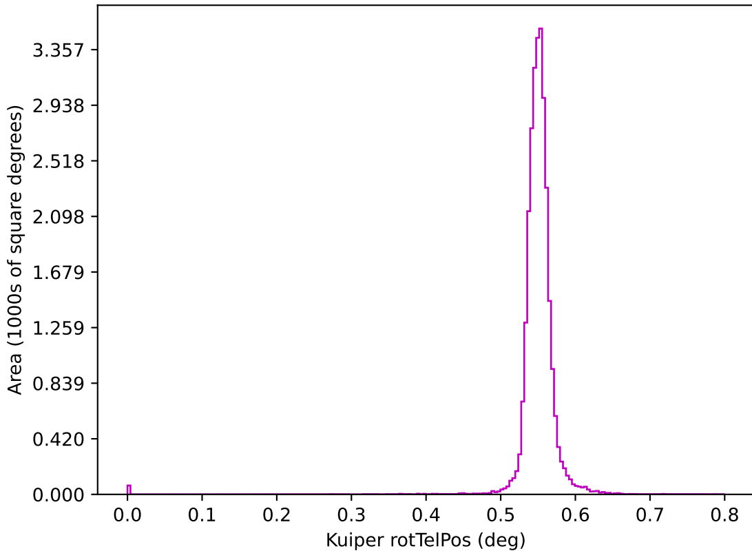
ddf_acor_sf20_lsf0_lsr0_v3.4_10yrs z: Kuiper rotTelPos
