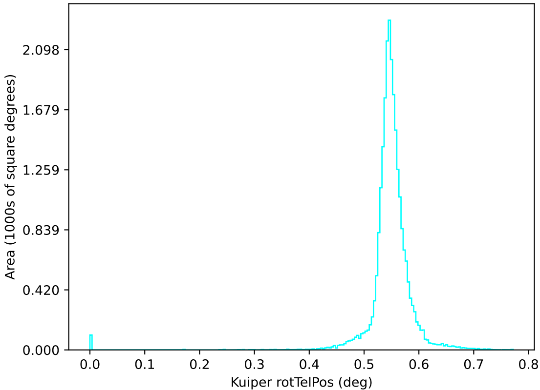
ddf_acor_sf20_lsf0_lsr0_v3.4_10yrs u: Kuiper rotTelPos
