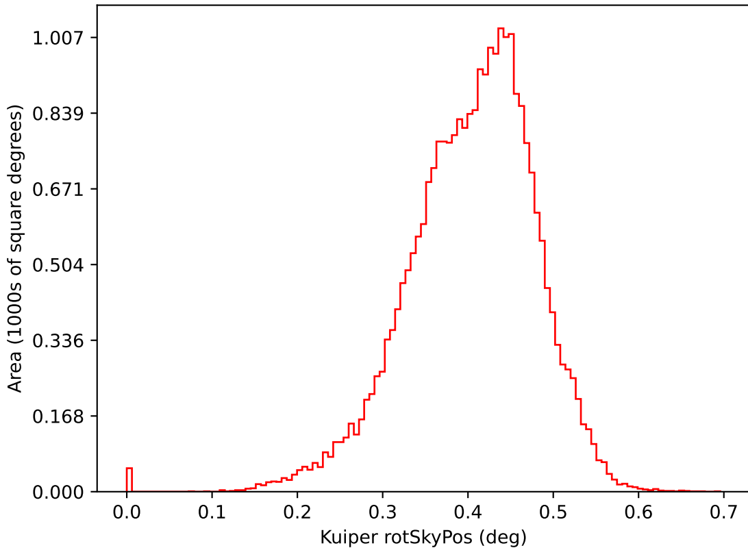
ddf_acor_sf20_lsf0_lsr0_v3.4_10yrs i: Kuiper rotSkyPos
