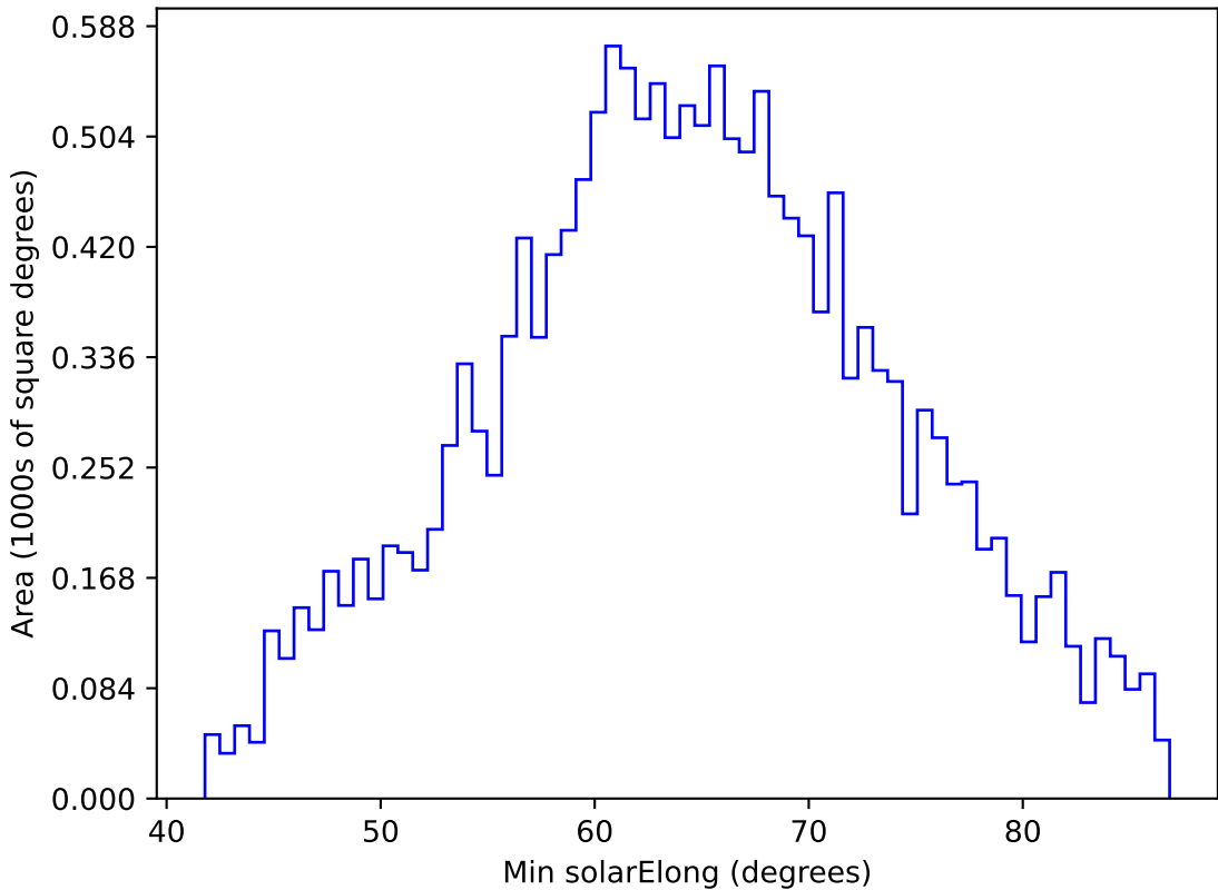
ddf_acor_sf20_lsf0_lsr0_v3.4_10yrs WFD y band: Min solarElong
